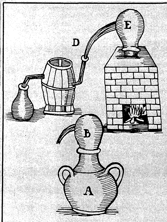
Eenvoudige destillatie-opstelling uit de achttiende eeuw. A is de eigenlijke destillatieketel. Vanaf de 'kop' (B en E) druppelt het destillaat naar het koelvat (bij D) en komt uiteindelijk uiterst links in het opvangvatje terecht.
